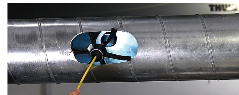
Inspection d'un conduit aérodynamique avec la caméra d'inspection connectée Wöhler SI 400.
